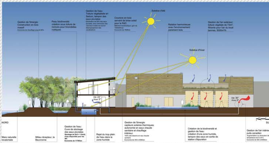
Architecture bioclimatique du bâtiment d'exploitation Coupe HQE
