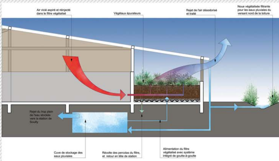
Traitement de l'air du hangar de stockage des boues par biofiltre végétalisé
