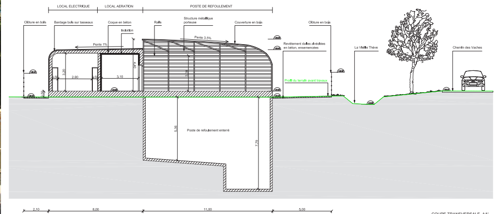
Coupe du poste technique PR7
